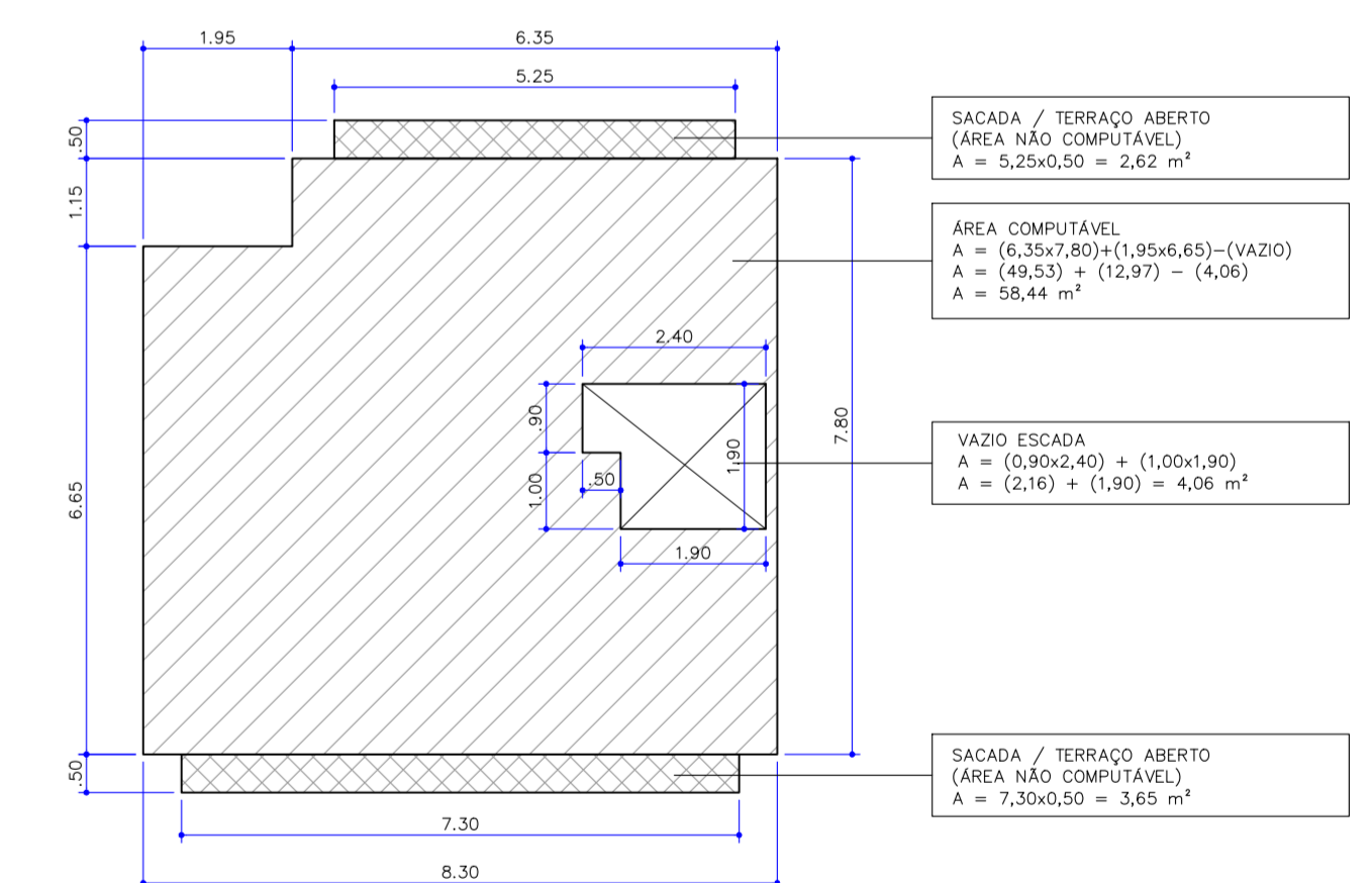
CASA TIPO C3 ESQUERDA PAV. TÉRREO ESC. 1:100
