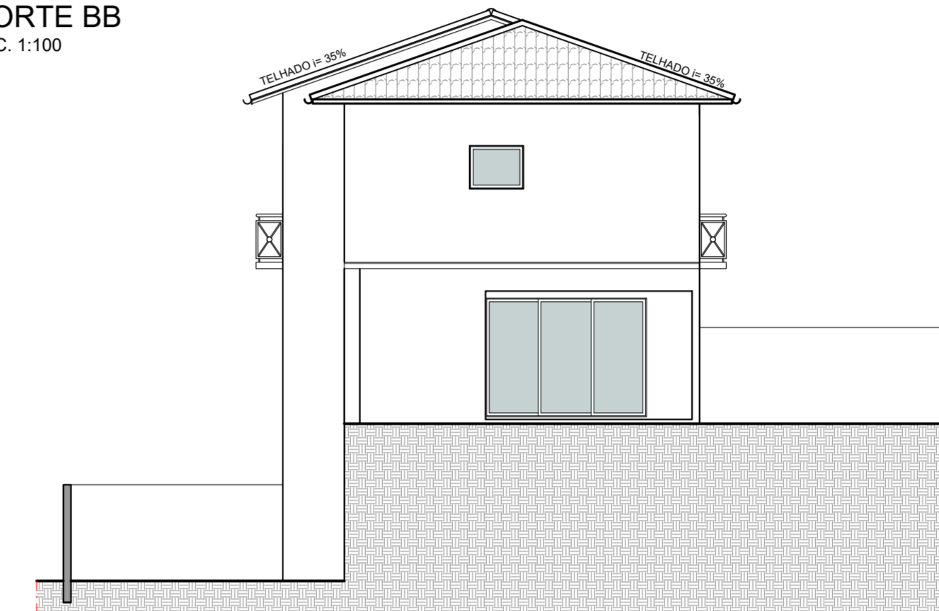
CASA TIPO C3 ESQUERDA (terreno em declive) ELEVÇÃO LATERAL ESC. 1:100
