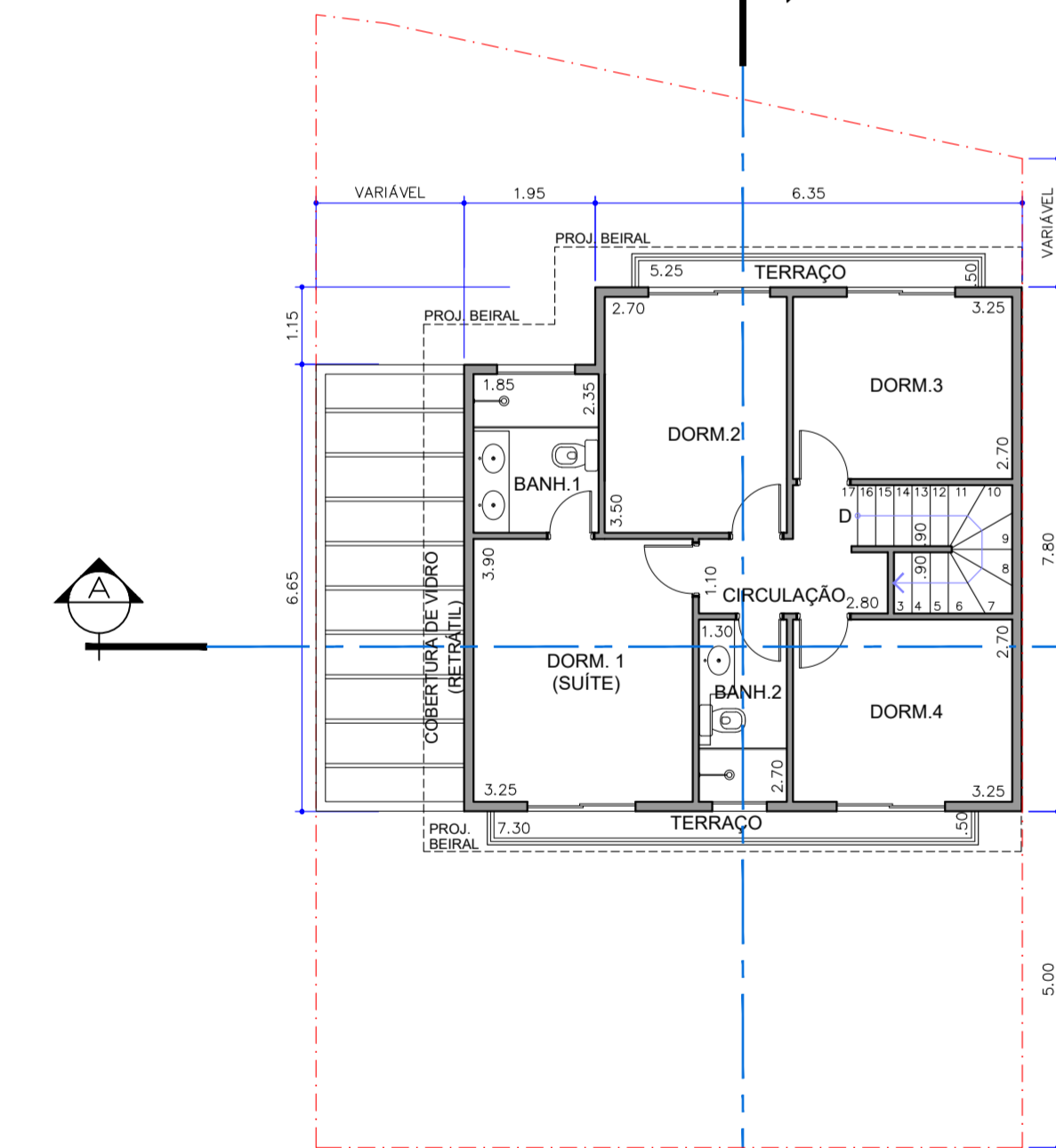
CASA TIPO C3 ESQUERDA (terreno em declive) PLANTA PAV. SUPERIOR ESC. 1:100 MODELO IMPLANTADO EM LOTES DE GEOMETRIA IRREGULAR
