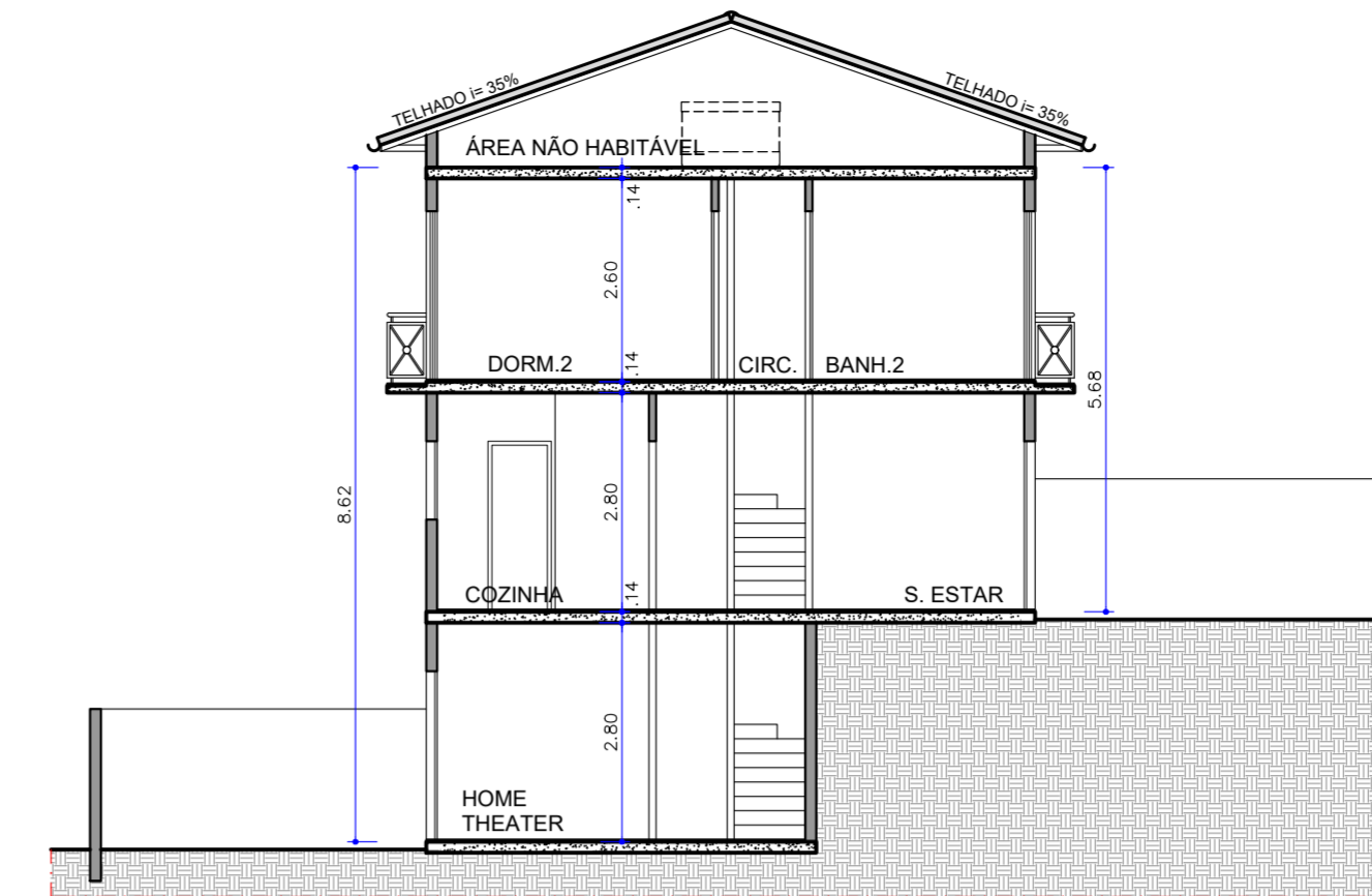
CASA TIPO C3 (terreno em declive) CORTE BB ESC. 1:100
