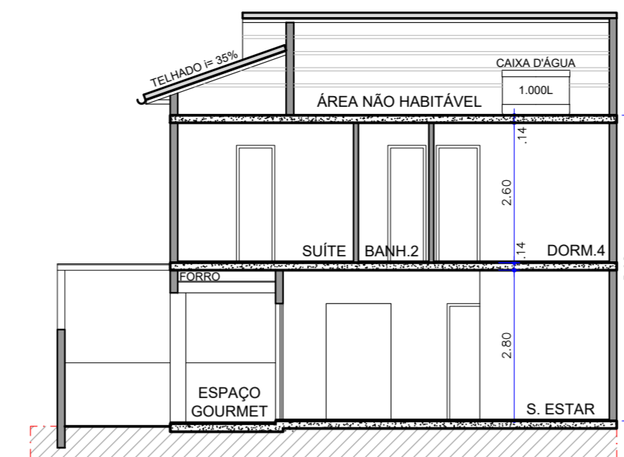
CASA TIPO C3 (terreno em declive) CORTE AA ESC. 1:100
