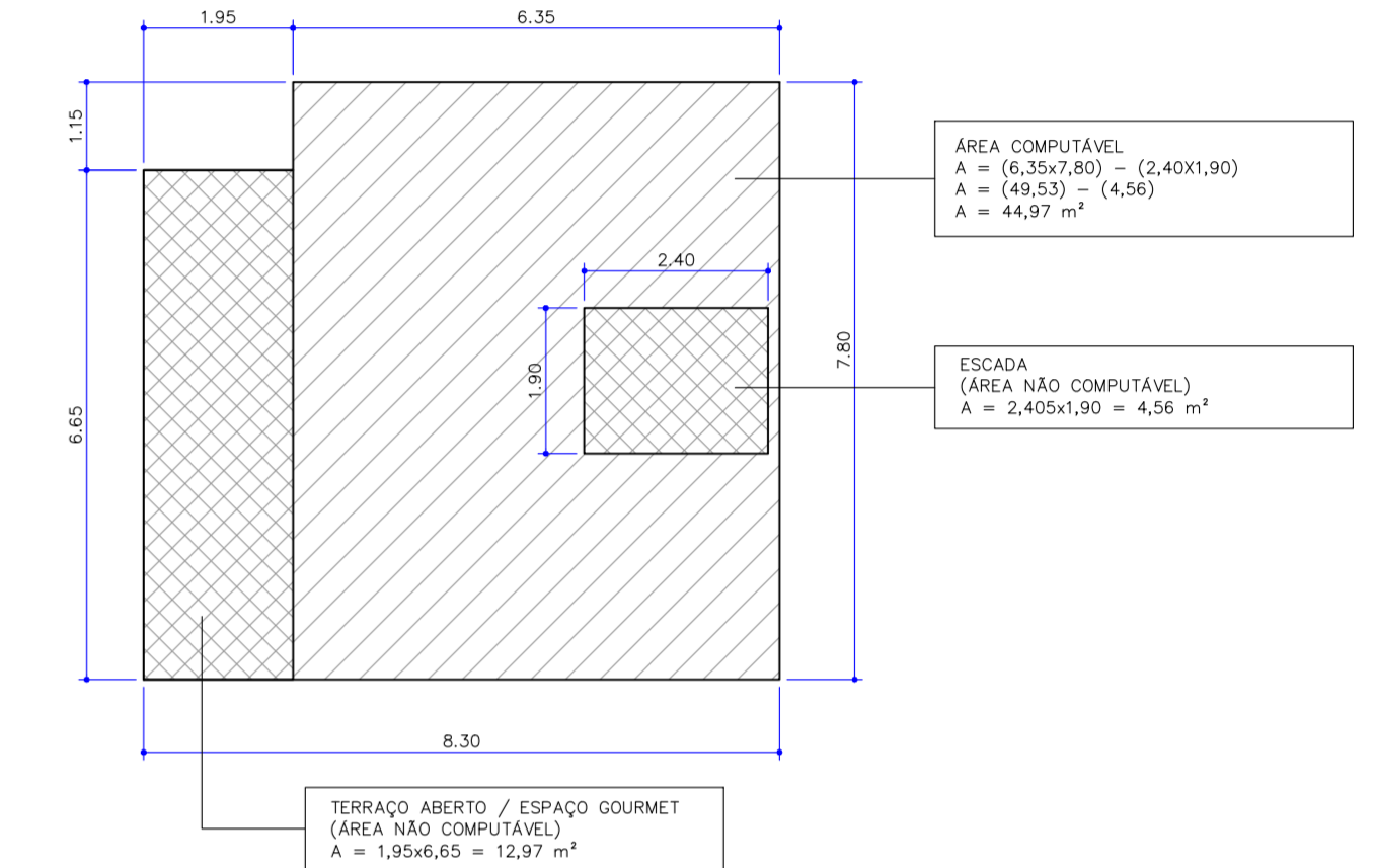
CASA TIPO C3 ESQUERDA PAV. INFERIOR ESC. 1:100
