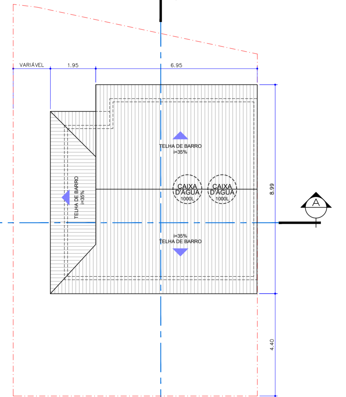
CASA TIPO C3 ESQUERDA (terreno em declive) PLANTA COBERTURA ESC. 1:100 MODELO IMPLANTADO EM LOTES DE GEOMETRIA IRREGULAR
