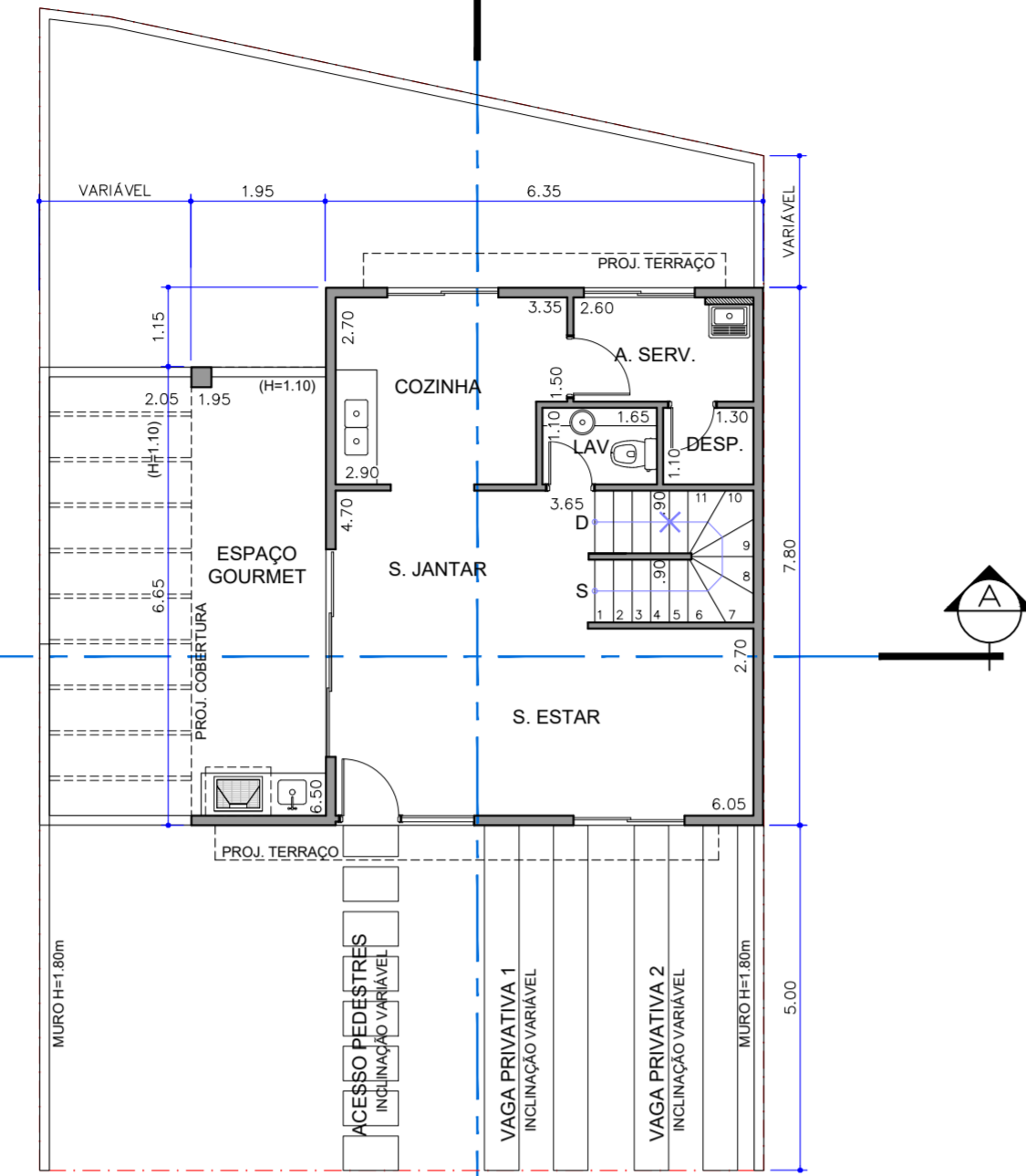
CASA TIPO C3 ESQUERDA (terreno em declive) PLANTA PAV. TÉRREO ESC. 1:100 MODELO IMPLANTADO EM LOTES DE GEOMETRIA IRREGULAR
