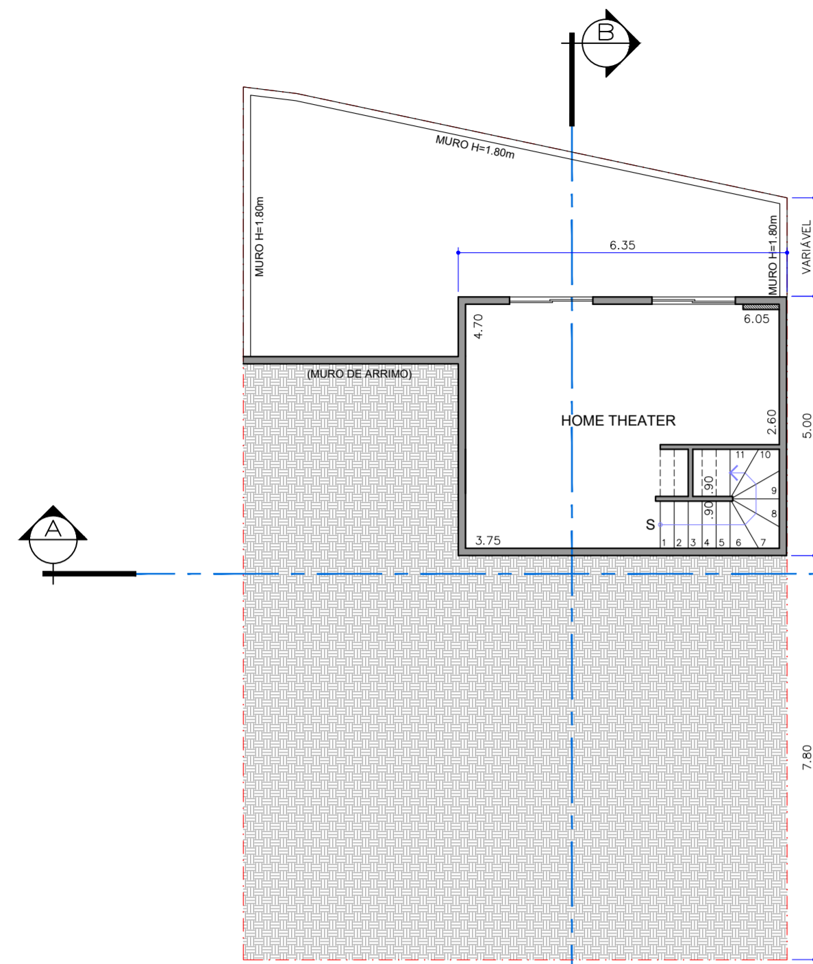
CASA TIPO C3 ESQUERDA (terreno em declive) PLANTA PAV. INFERIOR ESC. 1:100 MODELO IMPLANTADO EM LOTES DE GEOMETRIA IRREGULAR
